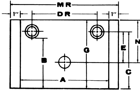
TYPE R DIE SET
