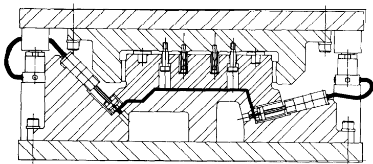
Automotive die . . . piercing
